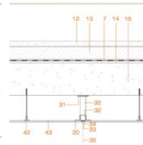
Cubierta tipo
