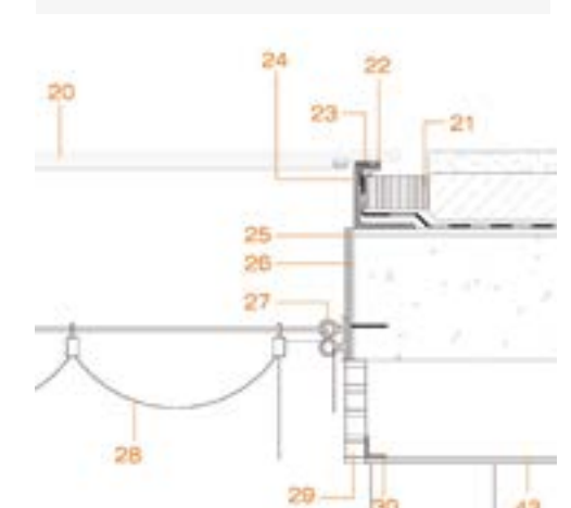
Encuentro de cubierta con lucernario
